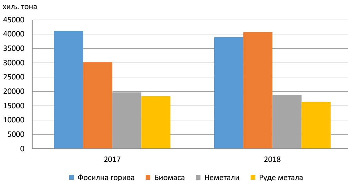
Граф. 1. Домаћи екстраховани ресурси према категоријама материјала
