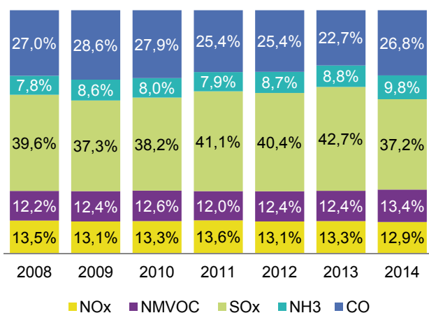
Емисије загађујућих материја, Република Србија, 2008–2014.
