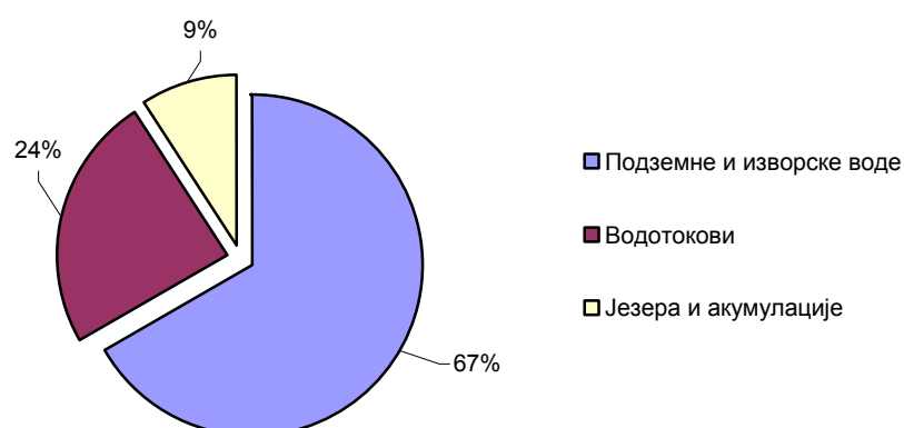
Графикон 1. Захваћена вода по врсти водозахвата у Републици Србији, 2015.
